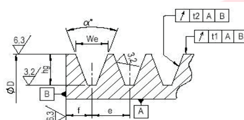
Dimensão TIPO DE PERFIL DO CANAL Z A B C D SPZ SPA SPB SPC 3V 5V 8V We ±0,2 9,7 12,7 16,3 22 32 9,7 12,7 16,3 22 8,9 15,2 25,4 f (polia Ferro) 9,85 11,35 13,15 17 23 9,5 11,35 13,15 17 9,45 13,6 19,7 f (polia Alumínio) 8,35 9,85 11,65 - - 8,35 9,85 11,65 - - - - e 12 15 19 25,5 37 12 15 19 25,5 10,3 17,5 28,6 hg 9 13,8 17,5 19,5 28 11 13,8 17,5 23,8 9 15,2 25,4 hg mín. 9 11,45 14,3 19,1 28 11 13,75 17,5 23,8 8,9 15,2 25,4 α ±0,5° 34° D≤80 D≤118 D≤190 D≤315 - D≤80 D≤118 D≤190 D≤315 - - - 36° - - - - D≤475 - - - - D≤90 - - 38° D>80 D>118 D>190 D>315 D>475 D>60 D>118 D>190 D>315 90<D≤150 D≤250 D≤400 40° - - - - - - - - - 150<D≤300 250<D≤400 400<D≤560 42° - - - - - - - - - D>300 D>400 D>560 Tolerância em e ±0,3 ±0,3 ±0,4 ±0,5 ±0,6 ±0,3 ±0,3 ±0,4 ±0,5 ±0,25 ±0,25 ±0,4 Soma dos desvios de e ±0,6 ±0,6 ±0,8 ±1 ±1,2 ±0,6 ±0,6 ±0,8 ±1 ±0,5 ±0,5 ±0,8 ØD mín. Recomendado 50 75 125 200 355 63 90 140 224 67 180 315
